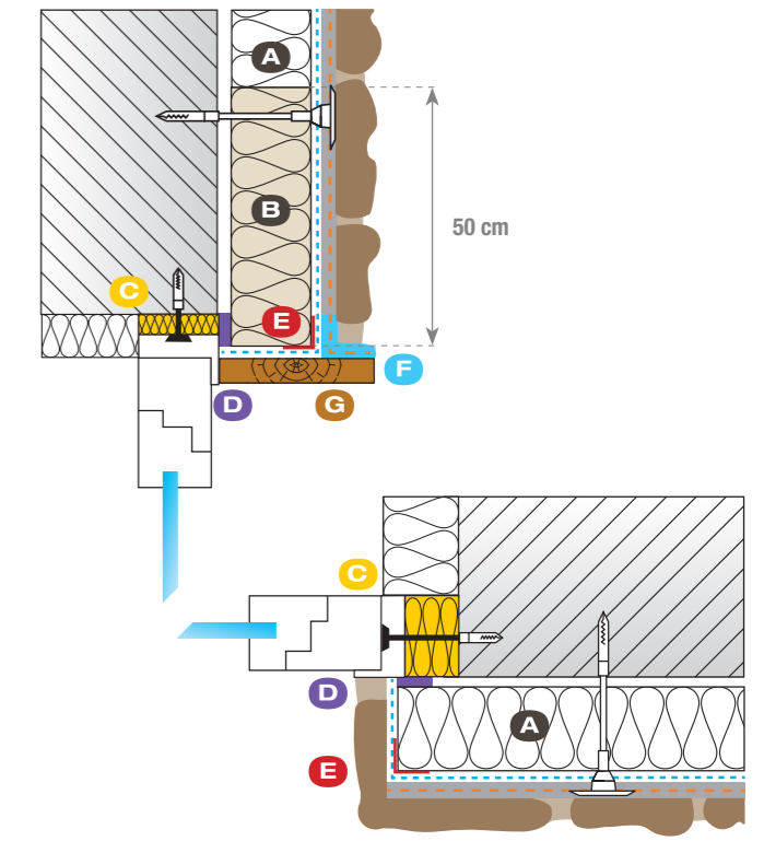
linteau de fenêtre avec poutre en bois
